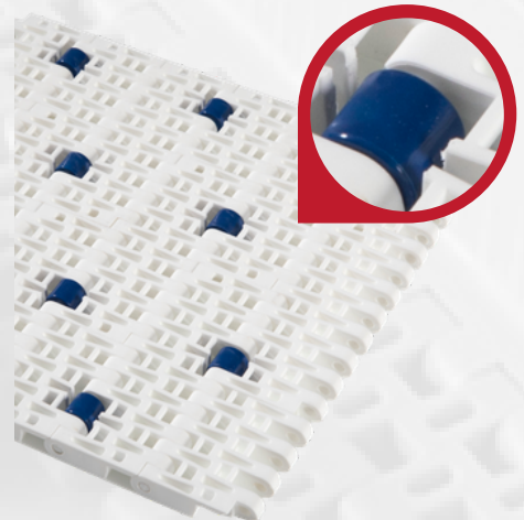
TAPIS PAS50.8/MDFGRT PAGE N°22
