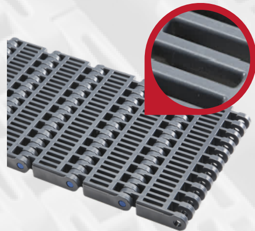
TAPIS PAS50.8/HPFG PAGE N°26
