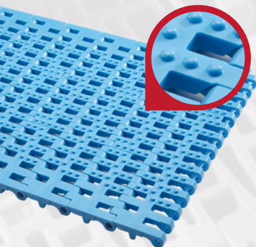
TAPIS PAS50.8/ECFGNT PAGE N°13
